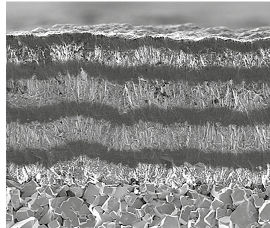
Vue en coupe d'un revêtement diamant multicouche breveté CemeCon. Une adhésion parfaite et une surface très lisse,
